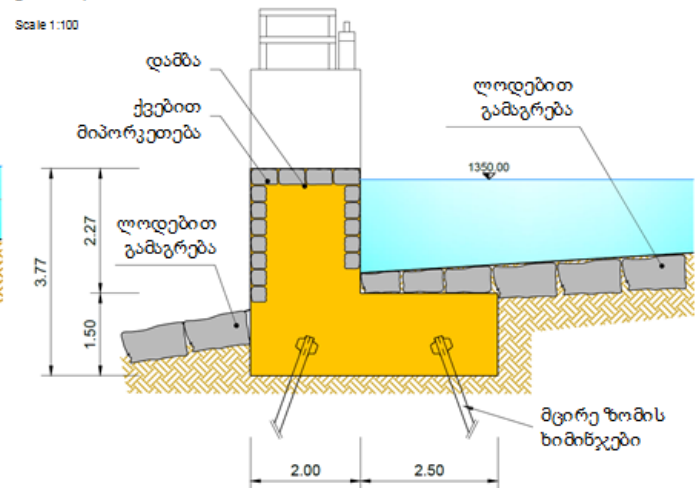
ჭრილი B-B
